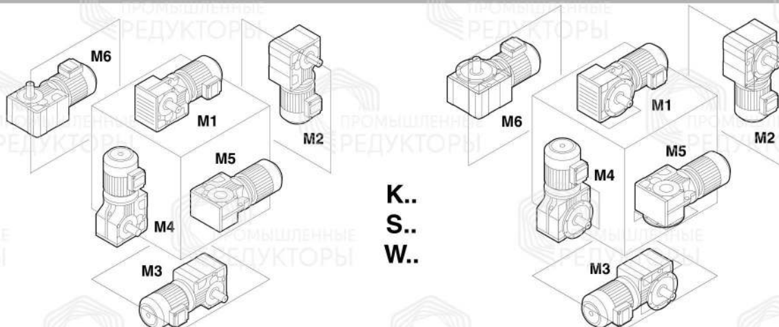
Рис. 8. Монтажные позиции M1...M6
